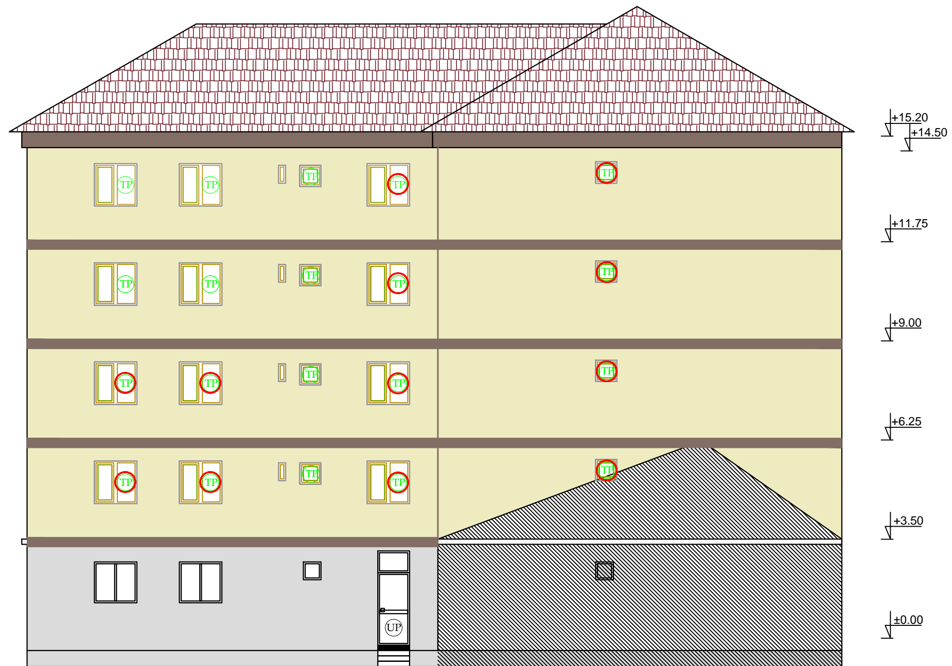
Fatada posteriora propusa Scara 1:100
